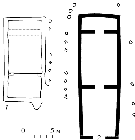
Рис. 8. 1 – обмерный план храма Аполлона Иетроса в Ольвии; 2 – схематический план мегарона в Фермосе
