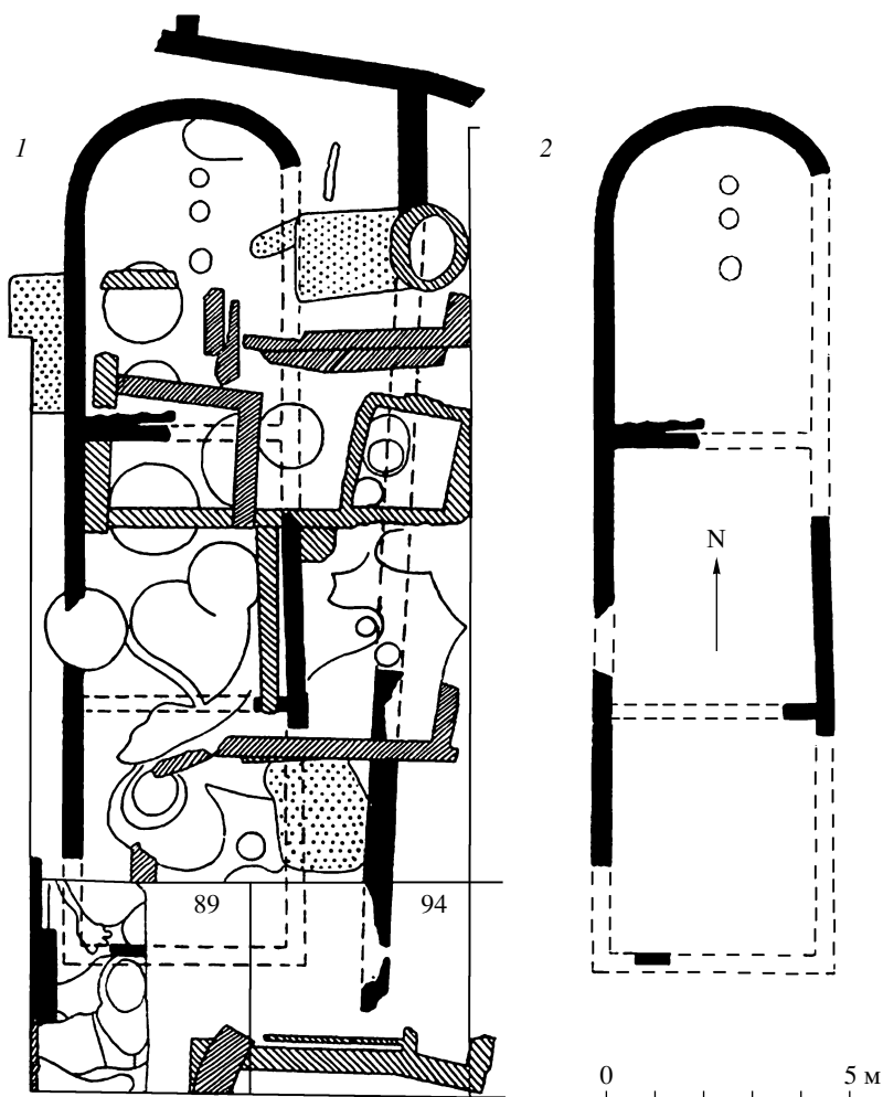
Рис. 2. Березань. Апсидальная постройка, раскопанная В.В. Лапиным. 1 – схематический план строительных остатков; 2 – реконструкция плана В.В. Лапина
