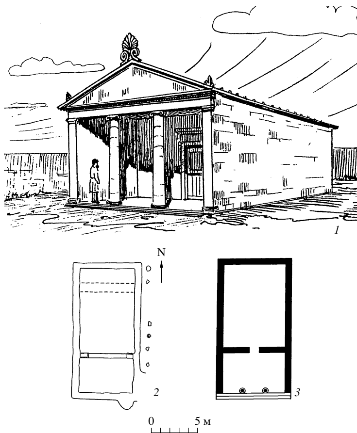
Рис. 6. Ольвия. Храм Аполлона Иетроса. 1 – общий вид; 2 – обмерный план; 3 – восстановление плана. Реконструкция С.Д. Крыжицкого
