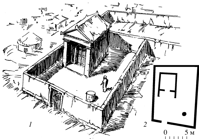
Рис. 4. Березань. Храм Афродиты. Реконструкция С.Д. Крыжицкого. 1 – общий вид; 2 – схематический план
