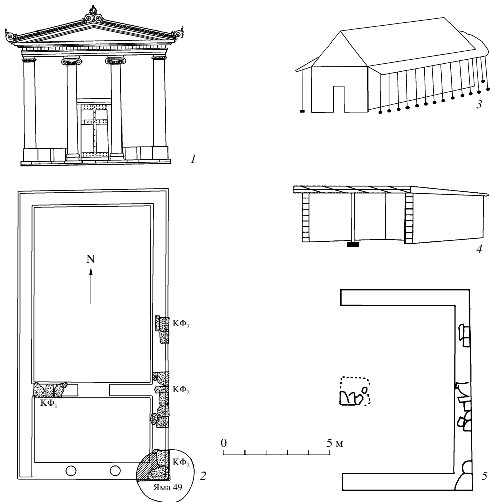
Рис. 9. Ольвия. 1 – реконструкция главного фасада «храма» Аполлона Дельфиния на Восточном теменосе А.Н. Карасева–И.Р. Пичикяна; 2 – реконструкция плана «храма» Аполлона Дельфиния А.Н. Карасева; 3 – реконструкция внешнего вида храма Аполлона Иетроса В.П. Яйленко; 4 – реконструкция общего вида «стои» В.П. Яйленко; 5 – реконструкция плана «стои» В.П. Яйленко
