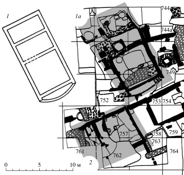
Рис. 3. Ольвия. «Мегаронные» постройки на раскопе экспедиции ЛОИА. 1 – реконструкция плана трехкамерной постройки Л.В. Копейкиной; 1а – схематический план строительных остатков трехкамерной постройки; 2 – схематический план строительных остатков двухкамерной постройки
