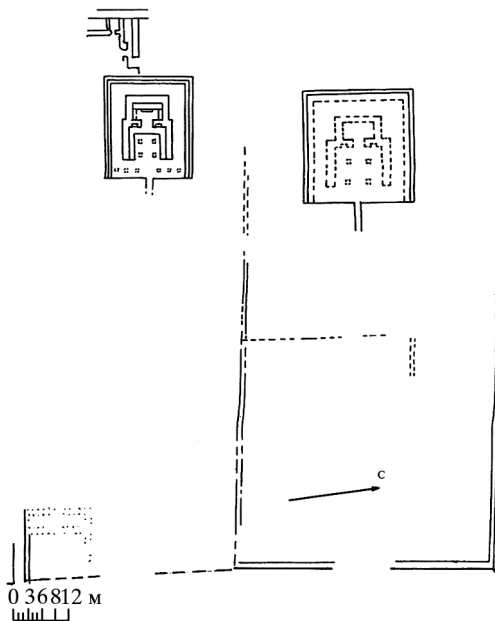
Рис. 7. Храмы Пенджикента. Планы
