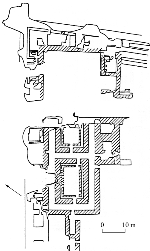
Рис. 5. Парфянское здание в Хурре. План
