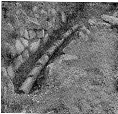
Рис. 9. Водопровод (в 700 м к западу-северо-западу от нимфея)
