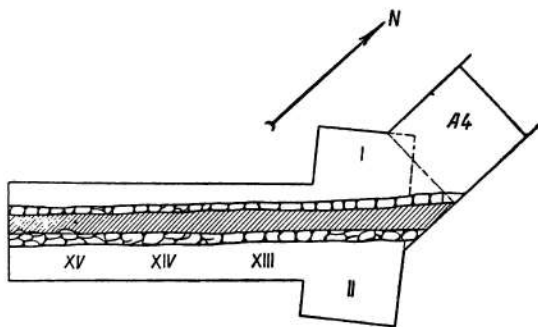
Рис. 5. План наружной оборонительной стены (раскопки 1935 г.)
